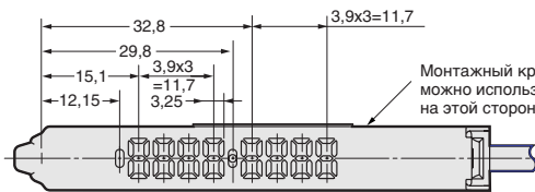
С установленным монтажным кронштейном
